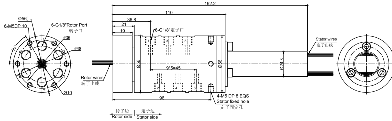
MKD61S-S56 尺寸图 6进6出G1/8"牙
