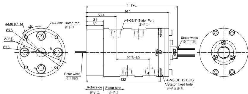
MKD43S-S06(S12,S18,S24,S36) 尺寸图 4进4出G3/8"牙+06~36路信号(2A)
